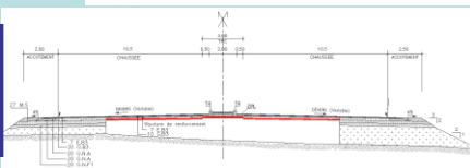
المقطع العرضي النموذجي
